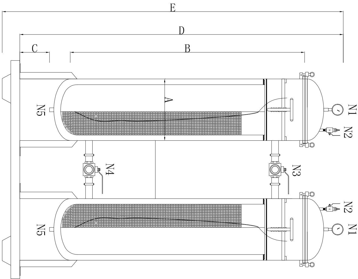
侧视图
