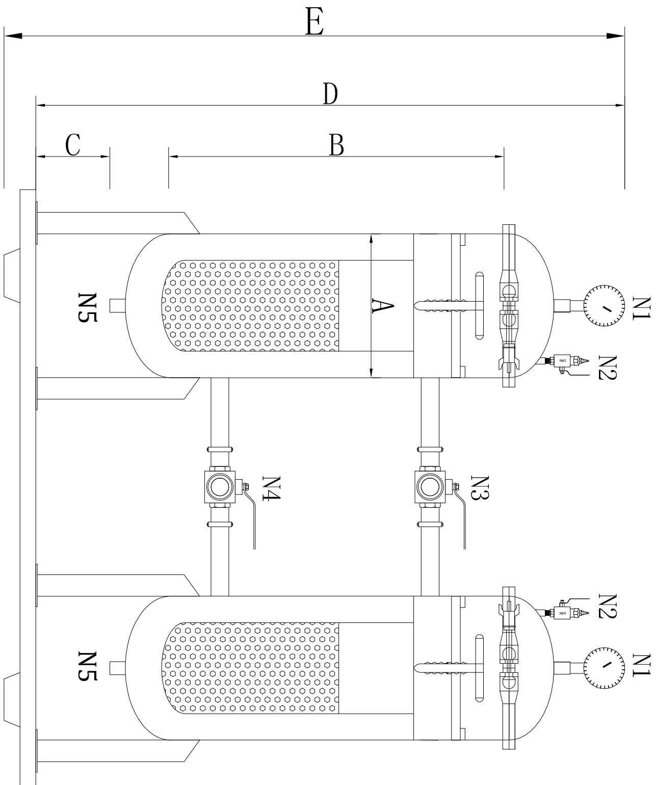
侧视图
