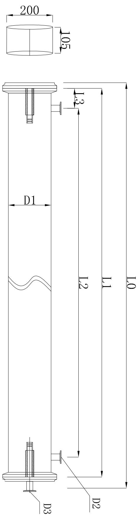
8英寸2芯膜壳图纸
