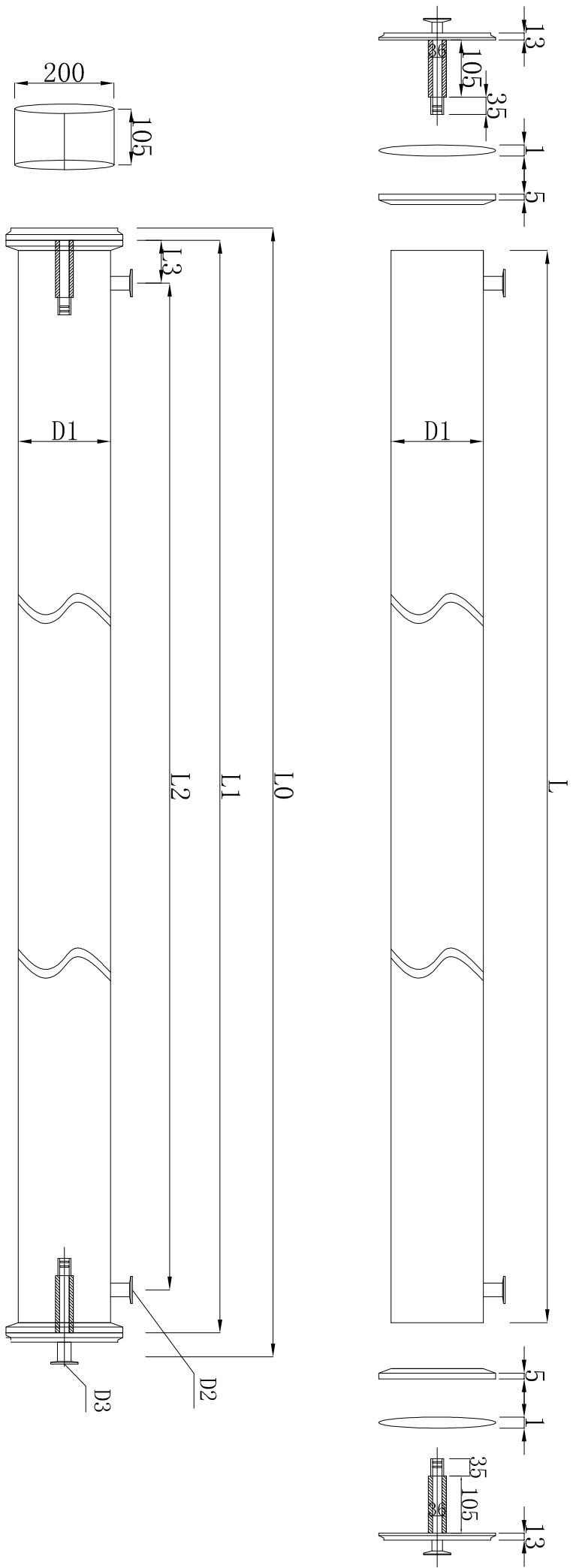
8英寸3芯膜壳图纸
