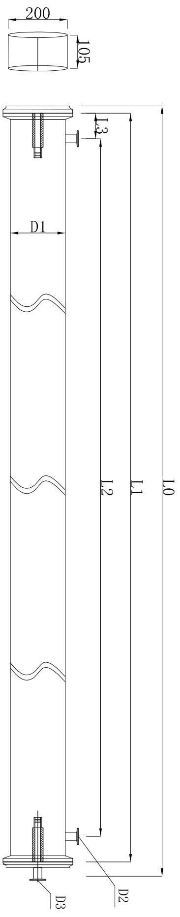
8英寸3芯膜壳图纸
