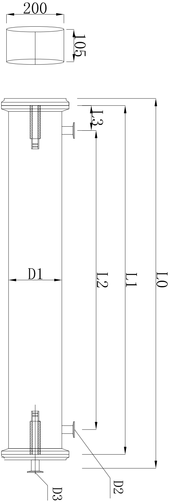
8英寸1芯膜壳图纸
